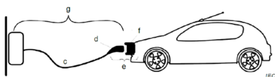
Kuva 2 Sähköajoneuvon lataaminen latausaseman rakenteeseen kuuluvalla latausjohdolla (IEC 61851-1)
