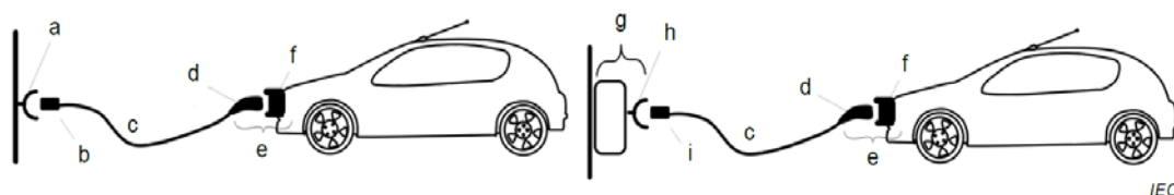
Kuva 1 Sähköajoneuvon lataaminen irrotettavalla latausjohdolla, joka ei ole latausaseman eikä ajoneuvon osa (IEC 61851-1)
